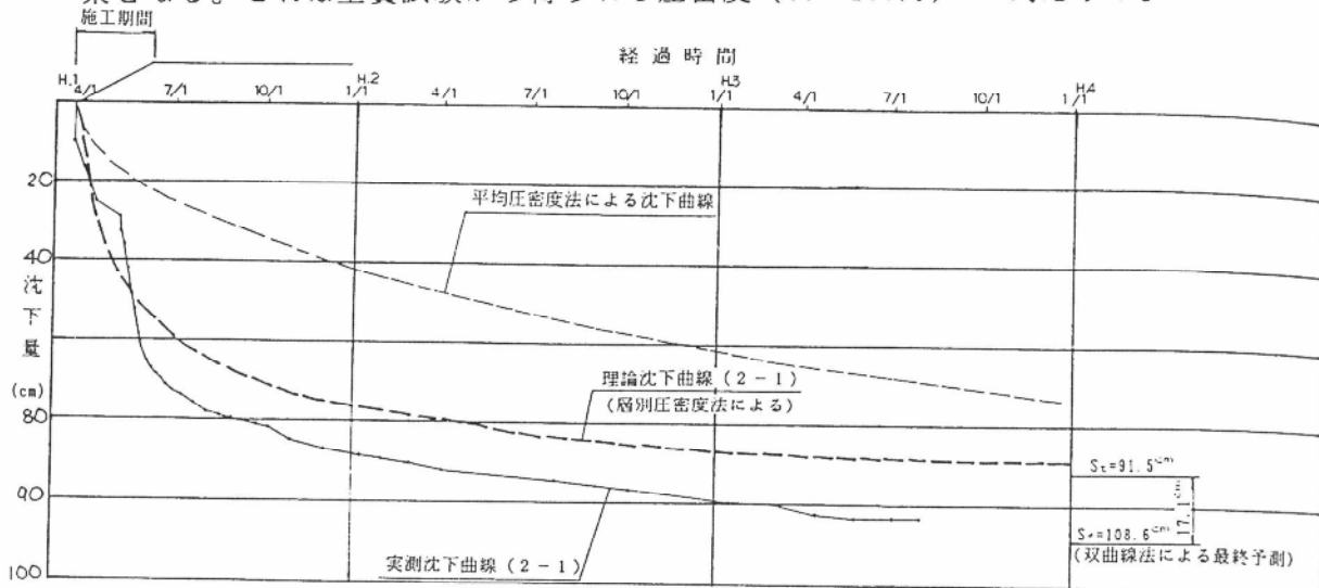
図-4 沈下量-沈下時間曲線
