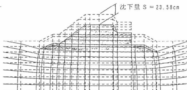
図-6 変形図(横断方向)
