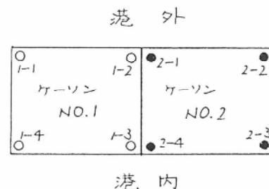
図-3 沈下観測点
