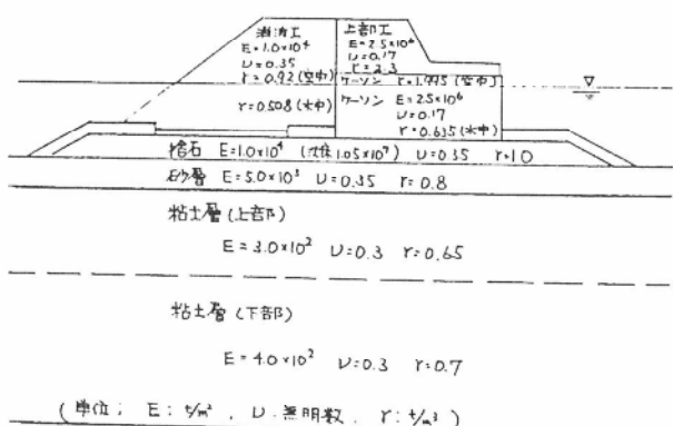
図-5 地盤及び防波堤の物性値
